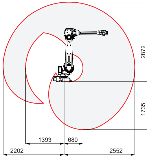
IRB 4600-40/2.55, 工作范围图例
